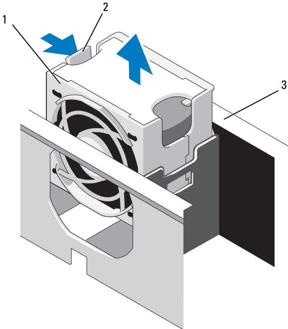
Abbildung 3-14. Entfernen und Installieren des Lüfters
