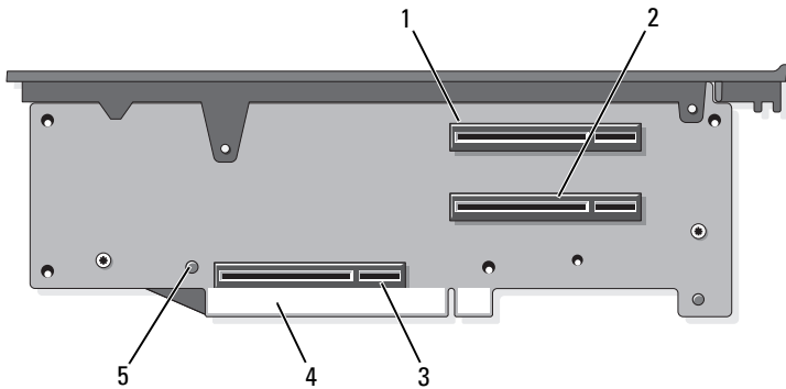
Abbildung 6-4. Komponenten der Steckkarte 1 für PCIe-Erweiterungskarten
