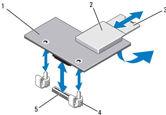
Abbildung 3-11. Entfernen und installieren der iDRAC6-Enterprise-Karte
