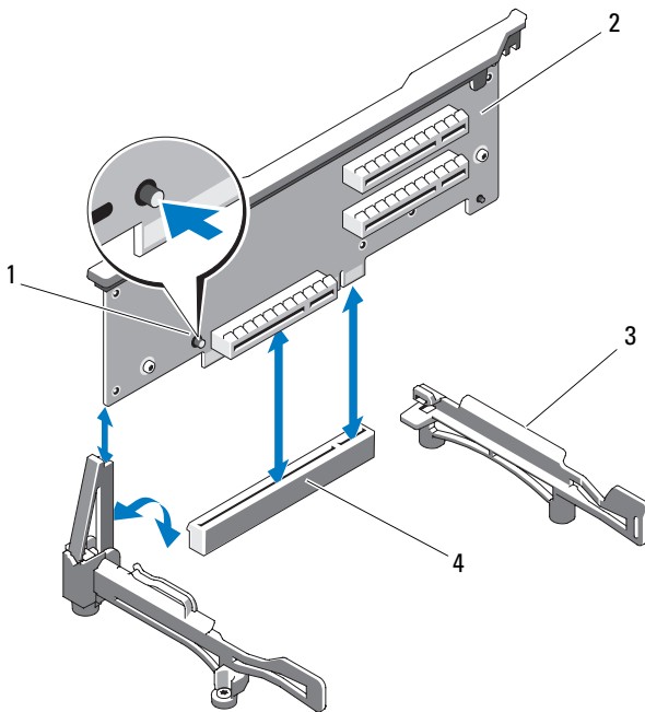
Abbildung 3-23. Erweiterungskarten-Steckkarte 1 entfernen und einsetzen
