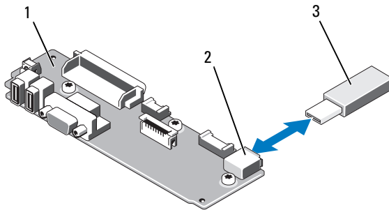
Abbildung 3-10. Entfernen oder Installieren des USB-Speichersticks
