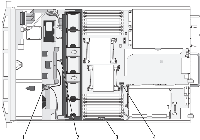
Abbildung 3-17. Führung des Kabels für das optische Laufwerk
