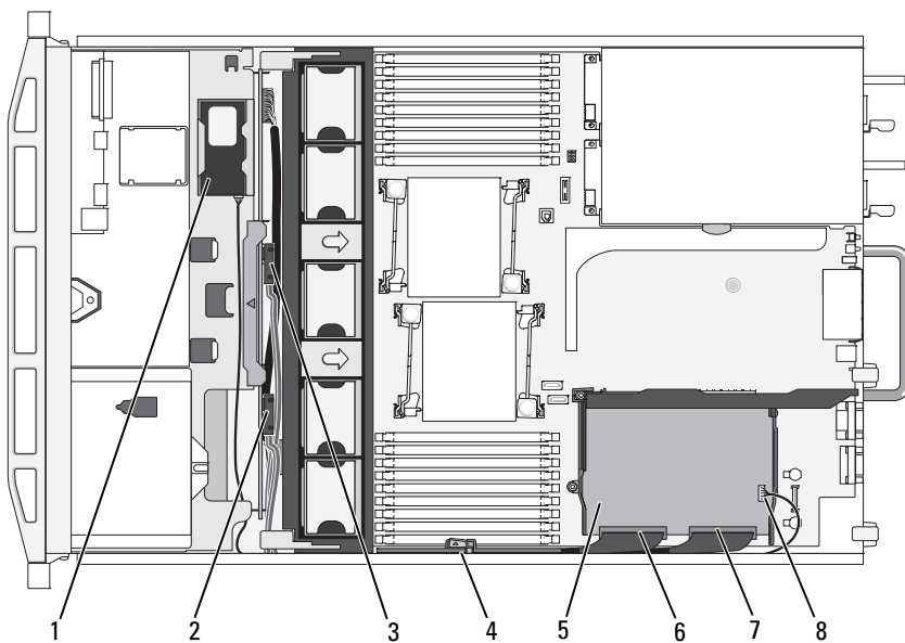
Abbildung 3-19. Verkabelung für die Speichercontrollerkarte
