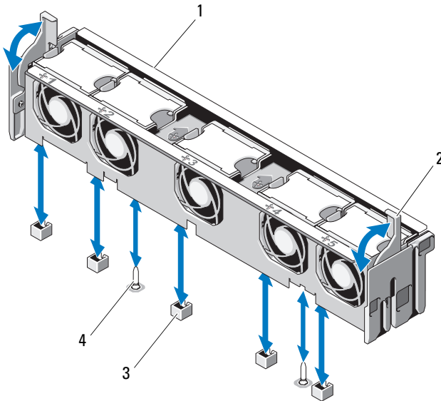
Abbildung 3-15. Prozessorlüfterhalterung entfernen und installieren
