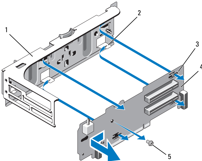
Abbildung 3-25. Steckkarte 2 entfernen und einsetzen
