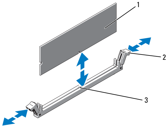
Abbildung 3-26. Installieren und Entfernen des Speichermoduls
