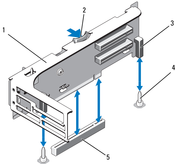
Abbildung 3-24. Erweiterungskarten-Steckkarte 2 entfernen und einsetzen
