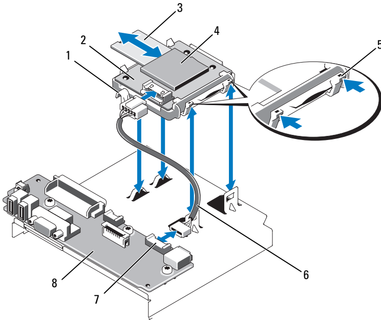
Abbildung 3-9. Entfernen oder Installieren des internen SD-Moduls
