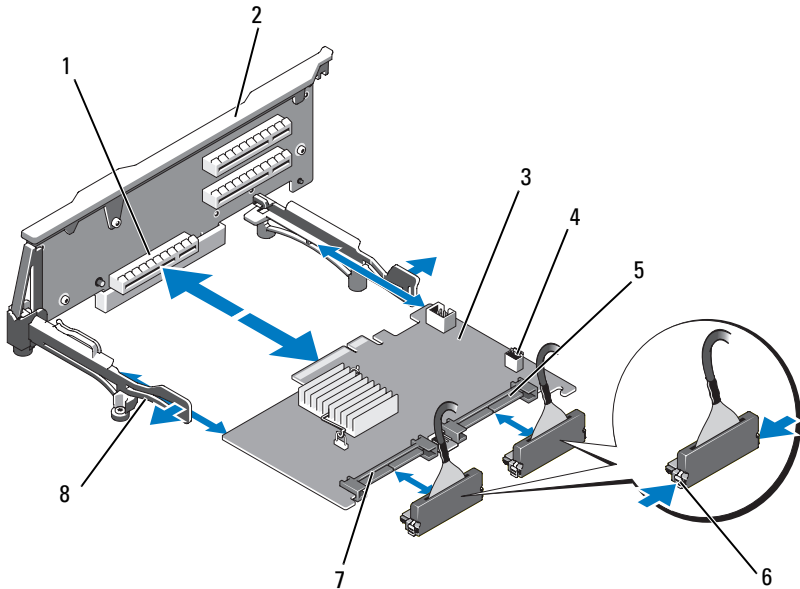
Abbildung 3-18. Installieren einer Speichercontrollerkarte
