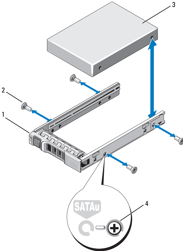
Abbildung 3-7. Installieren des Diskettenlaufwerks im Laufwerkträger
