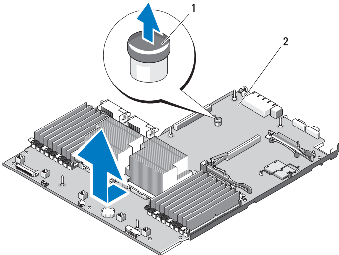
Abbildung 3-34. Systemplatine entfernen
