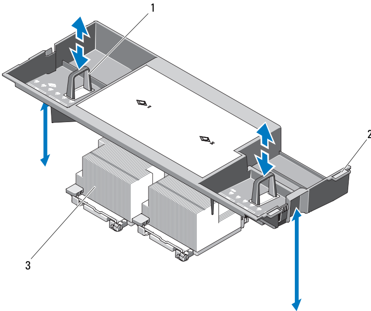
Abbildung 3-13. Kühlgehäuse entfernen und installieren
