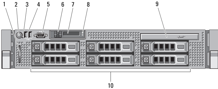
Abbildung 1-1. Funktionsmerkmale und Anzeigen auf der Vorderseite
