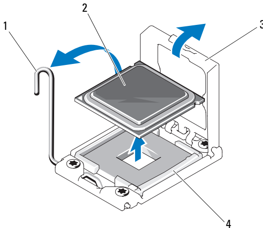
Abbildung 3-28. Entfernen des Prozessors
