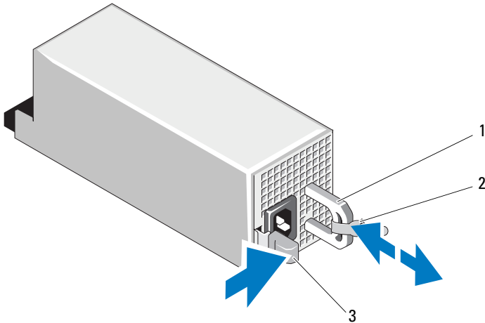
Abbildung 3-8. Netzteil entfernen und installieren
