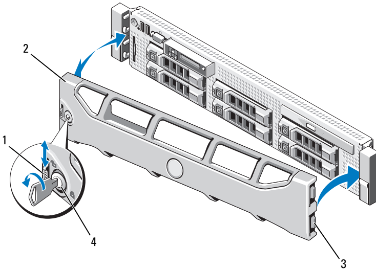
Abbildung 3-2. Abnehmen der Frontverkleidung
