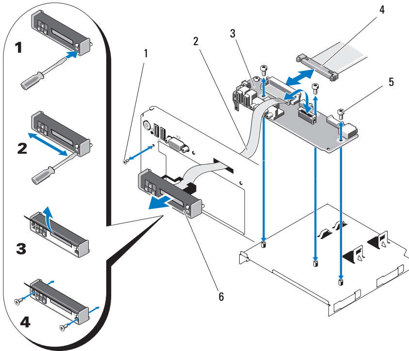
Abbildung 3-32. Bedienfeldplatine entfernen und installieren
