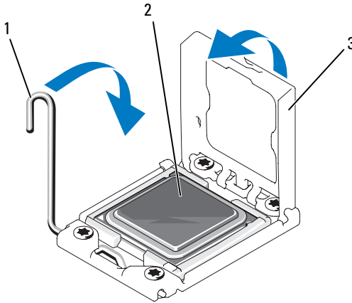
Abbildung 3-30. Schließen der Prozessorabdeckung
