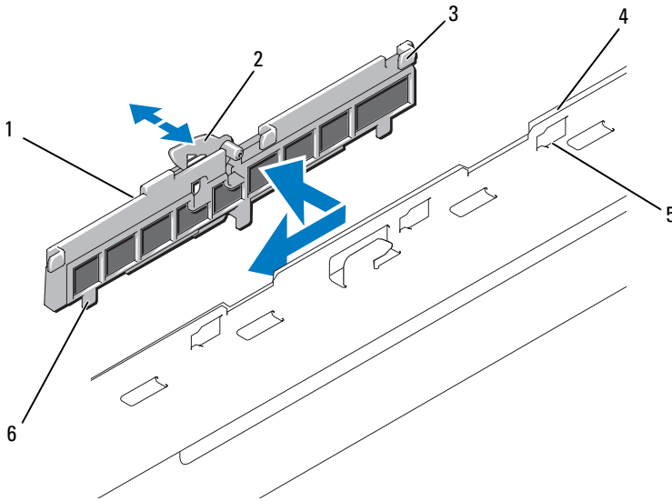
Abbildung 3-21. Entfernen und Installieren der Kabelhalteklammer
