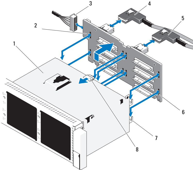
Abbildung 3-33. SAS-Rückwandplatine entfernen und installieren
