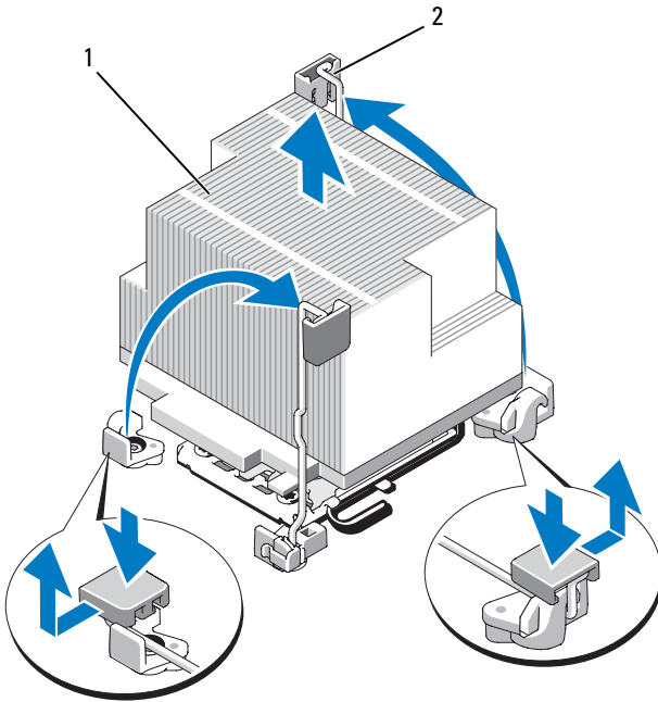
Abbildung 3-27. Kühlkörper installieren und entfernen
