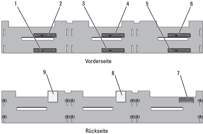
Abbildung 6-3. SAS-Rückwandplatine (6 Sockel)
