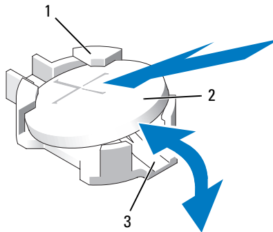
Abbildung 3-31. Systembatterie austauschen
